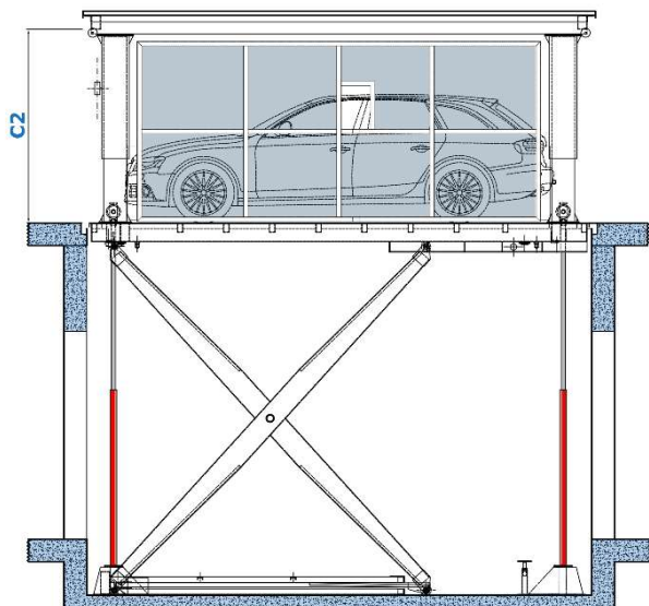
Vista in sezione - ALTO
